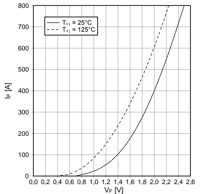
Durchlaßkennlinie der Diode-Wechsler. (typisch) forward characteristic of diode-inverter (typical) I_F = f(V_F)
