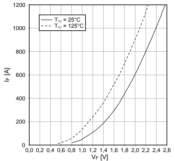
Durchlaßkennlinie der Diode-Wechselr. (typisch) forward characteristic of diode-inverter (typical) I_F = f(V_F)
